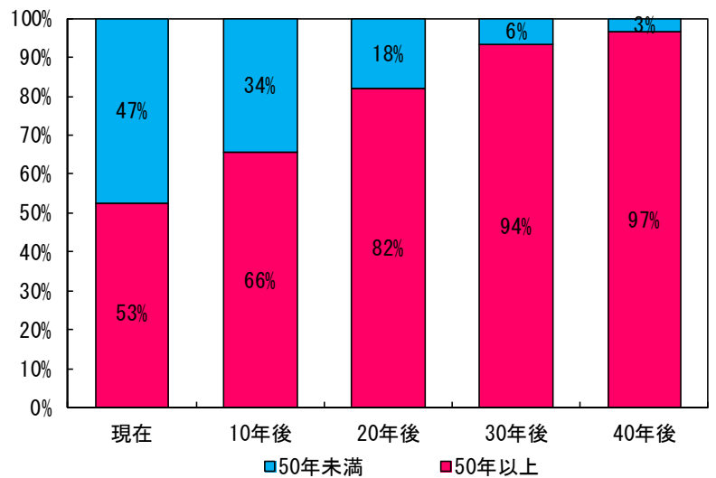
図-3.5 架設後50年以上の橋梁割合推移
